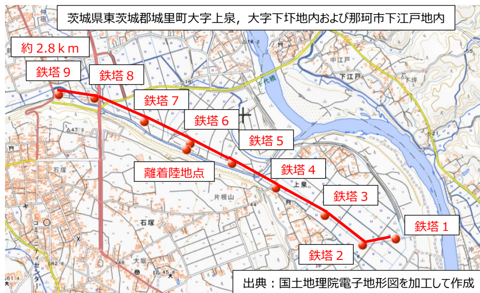
飛行経路図
